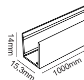
Monteringsskinne - 1m Art. nr. AS-NMT1312A-1000
