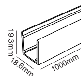
Monteringsskinne - 1m Art. nr. AS-NM3D1515A2-1000
