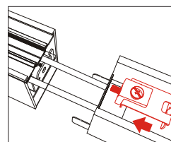
Monter fast Gearlink til armatur
