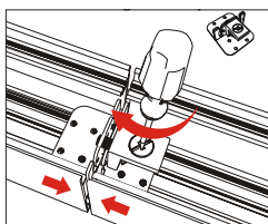
Benytt skrujern for å feste Gearlink til neste armatur
