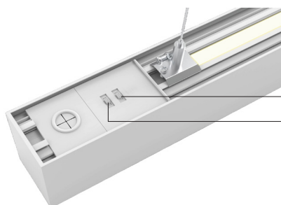
Opplys (av/på) Colour Switch (3000K/4000K)
