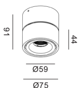
Glow 59
